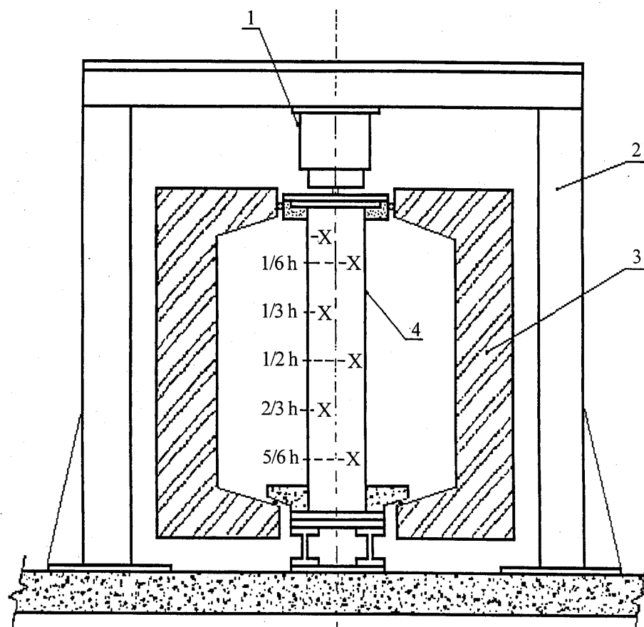
Рисунок А.7 – Схематичне зображення зразка навантаженої колони, встановленої у печі
